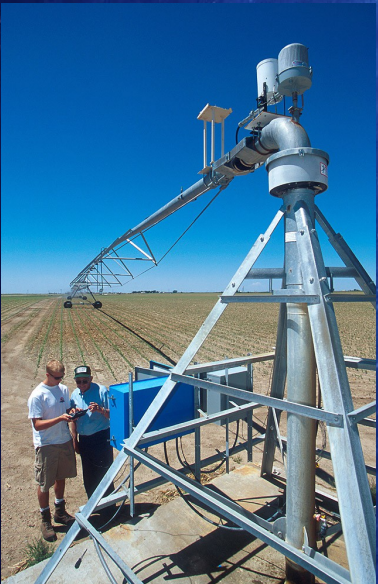
Rampe d'arrosage sur pivot
